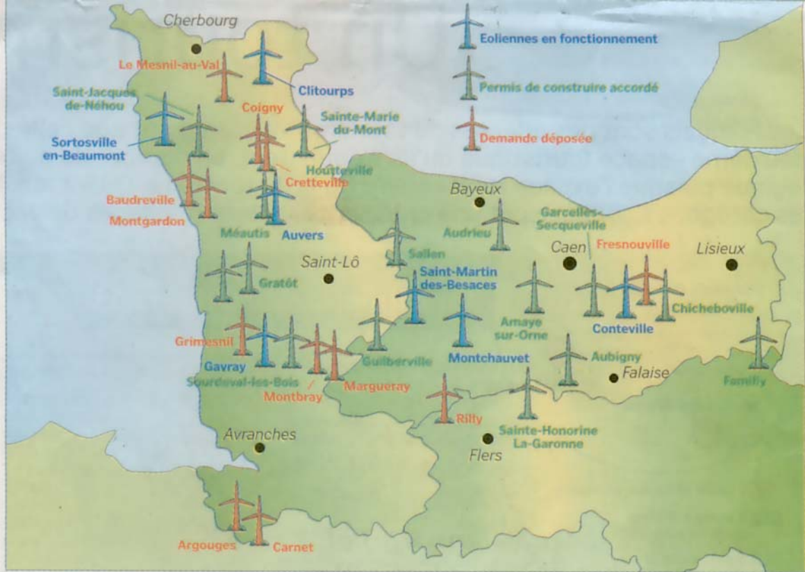
Le parc éolien de Sortosville-en-Beaumont près de Barneville-Carteret a vu le jour en 2004. C'est le premier qui a été construit en Basse-Normandie.
